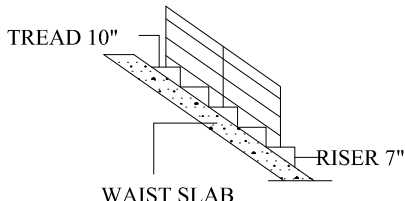
STAIRCASE DETAILS (N.T.S.)
