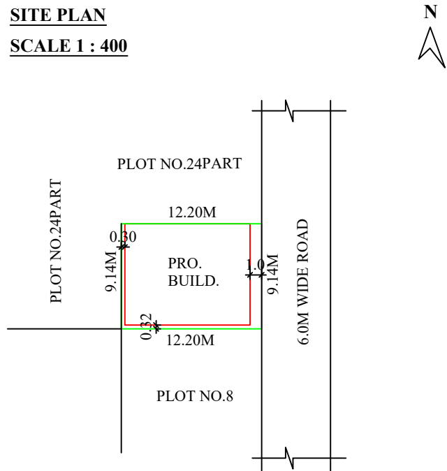
SITE EXTENT
