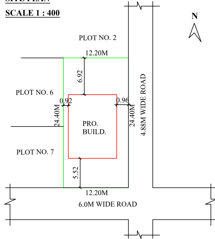
SITE EXTENT
