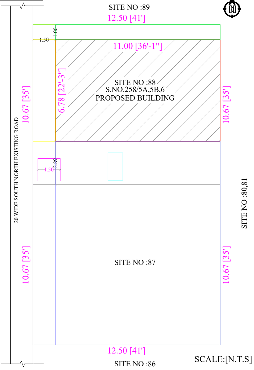
SITE PLAN :
