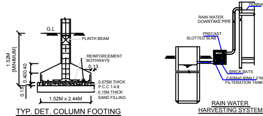
TYP. DET. COLUMN FOOTING
