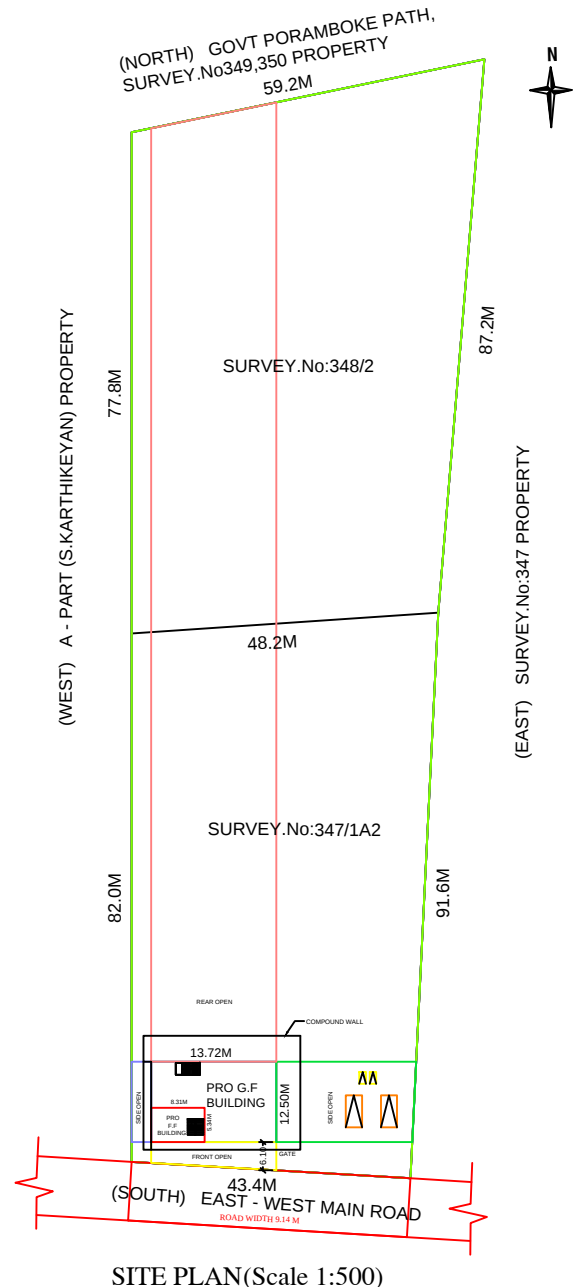
SITE PLAN(Scale 1:500)
