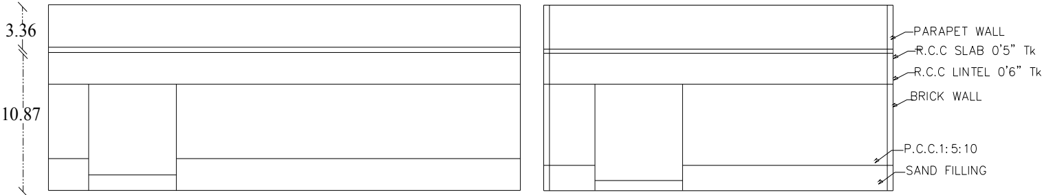
ELEVATION
