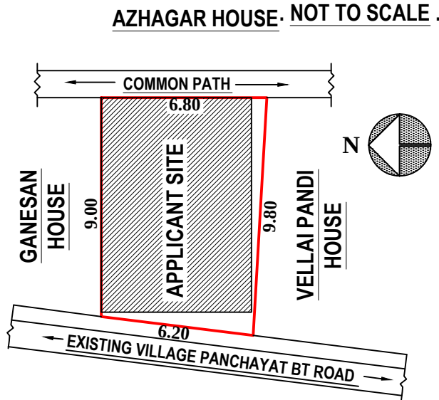
. SITE PLAN .
