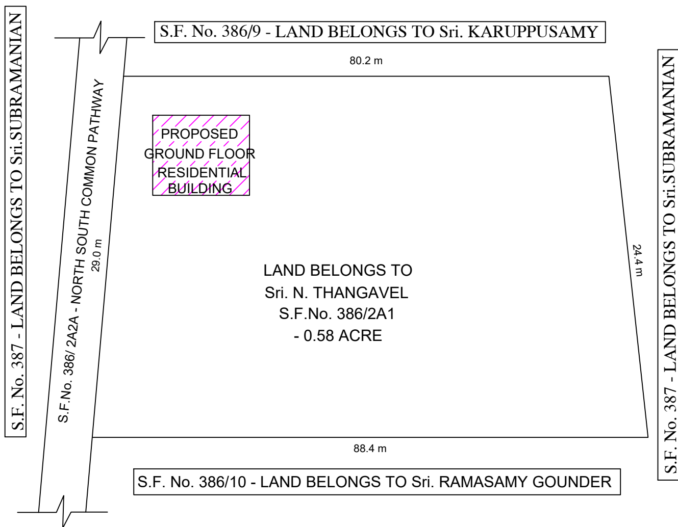
SITE PLAN SCALE : - NTS
