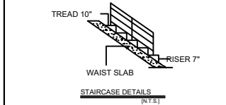
STAIRCASE DETAILS (N.T.S.)
