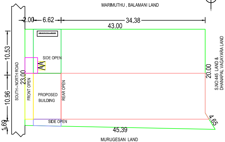
SITE PLAN : (SCALE 1:400)
