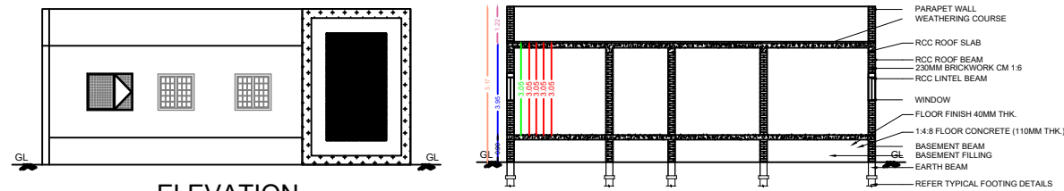
SECTION A-B
