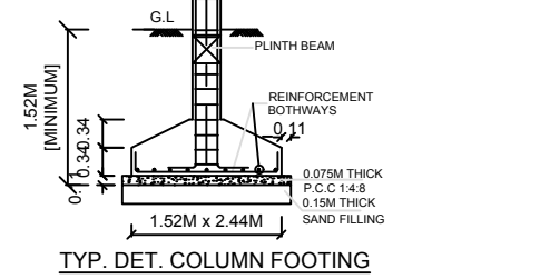
TYP. DET. COLUMN FOOTING
