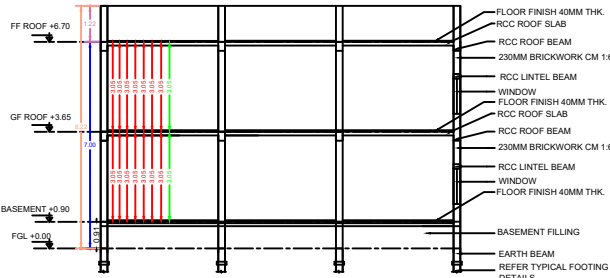
② SECTION A-B
