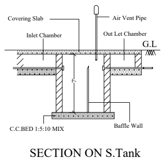
SECTION ON S.Tank (N.T.S.)
