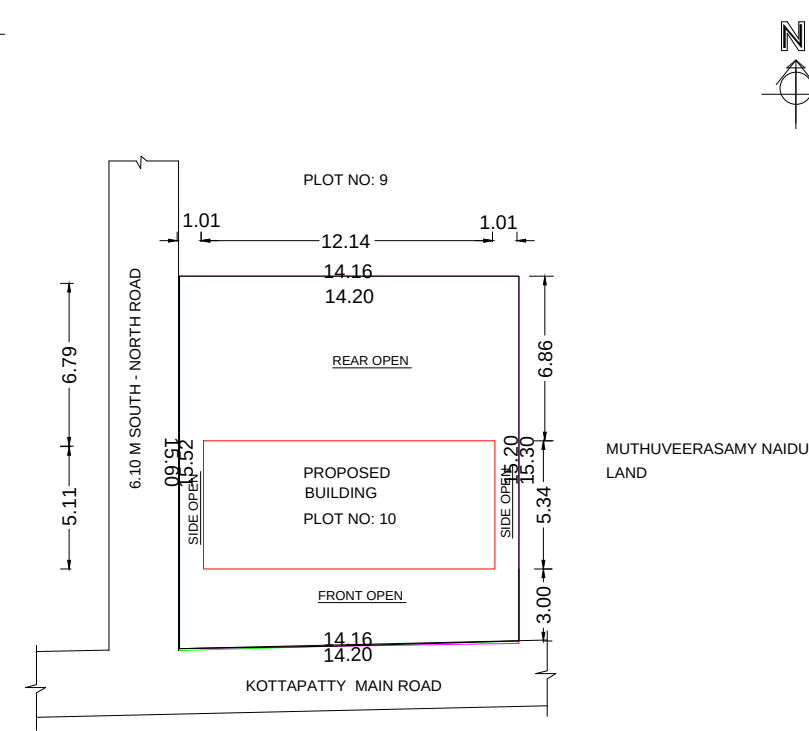
SITE PLAN : (SCALE 1:400)
