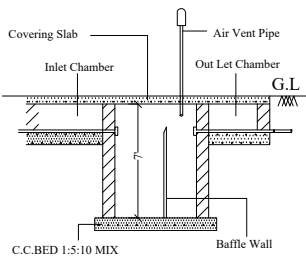
SECTION ON S.Tank (N.T.S.)
