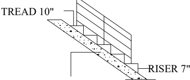
STAIRCASE DETAILS (N.T.S.)
