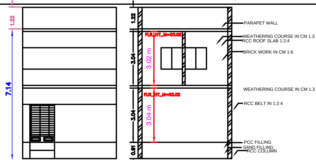
ELEVATION SECTIONNON-"AA"&"BB"
