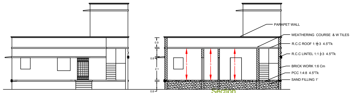
ELEVATION
