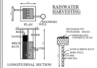
LONGITUDINAL SECTION
