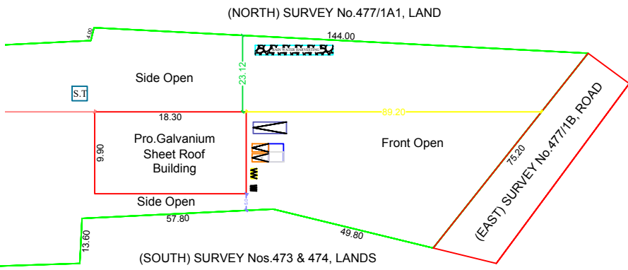
SITE PLAN (SCALE 1:400)
