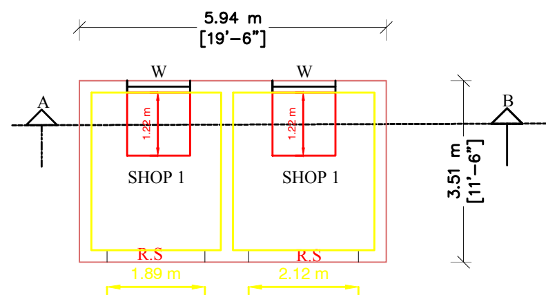
PLAN ( SCALE 1 : 100 )
