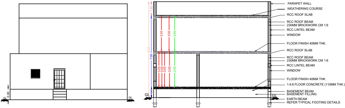
ELEVATION
