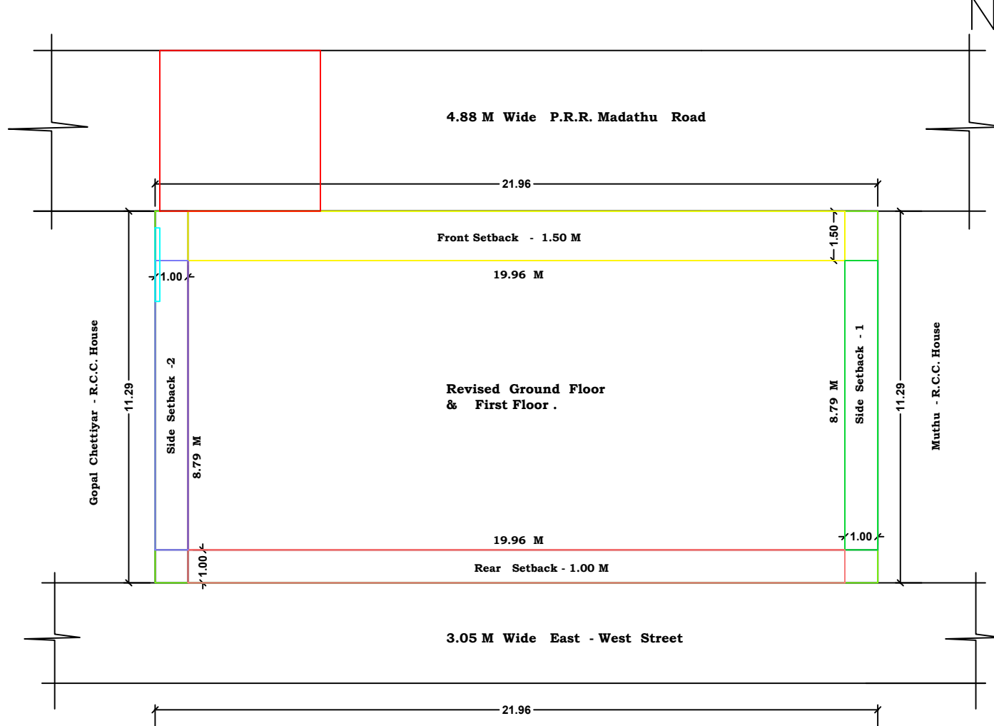
SITE PLAN 1:100
