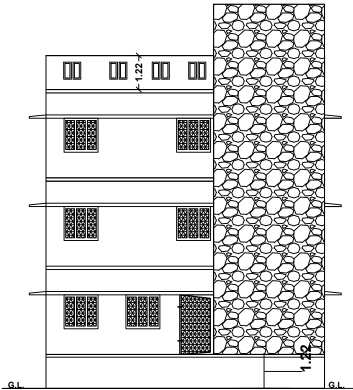
ELEVATION
