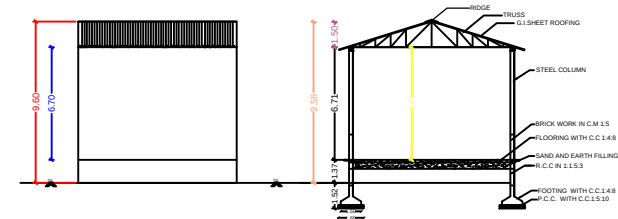
ELEVATION
