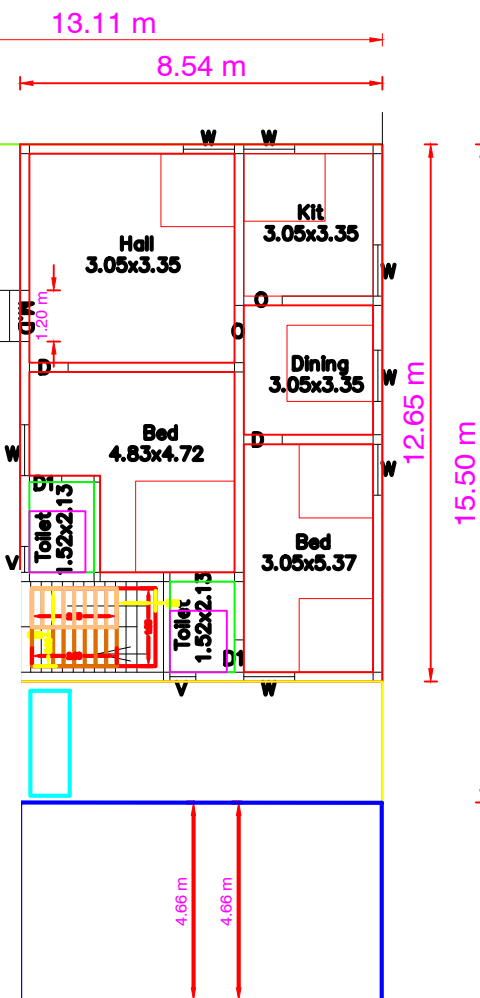
ROUND FLOOR(Pro.)
