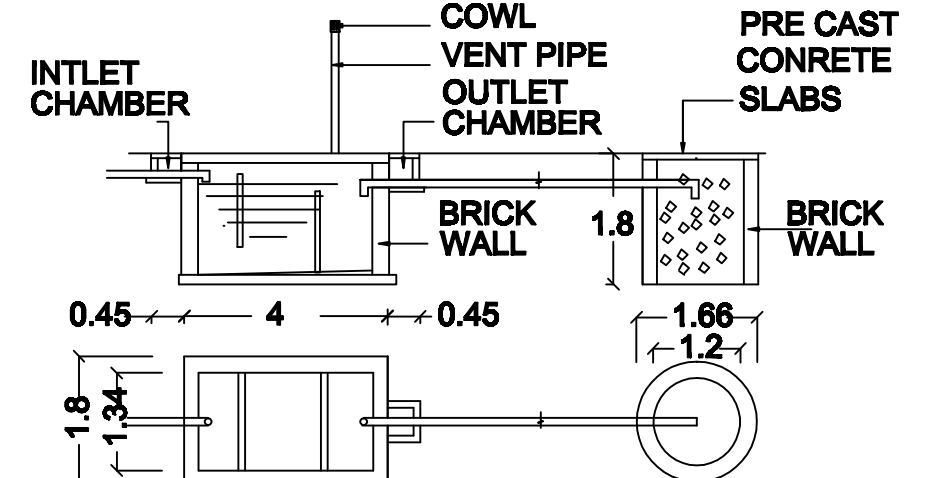
SEPTIC TANK & SOAK PIT (N.T.S)
