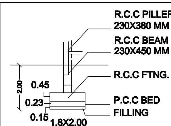
FOUNDATION DETAILS (N.T.S)
