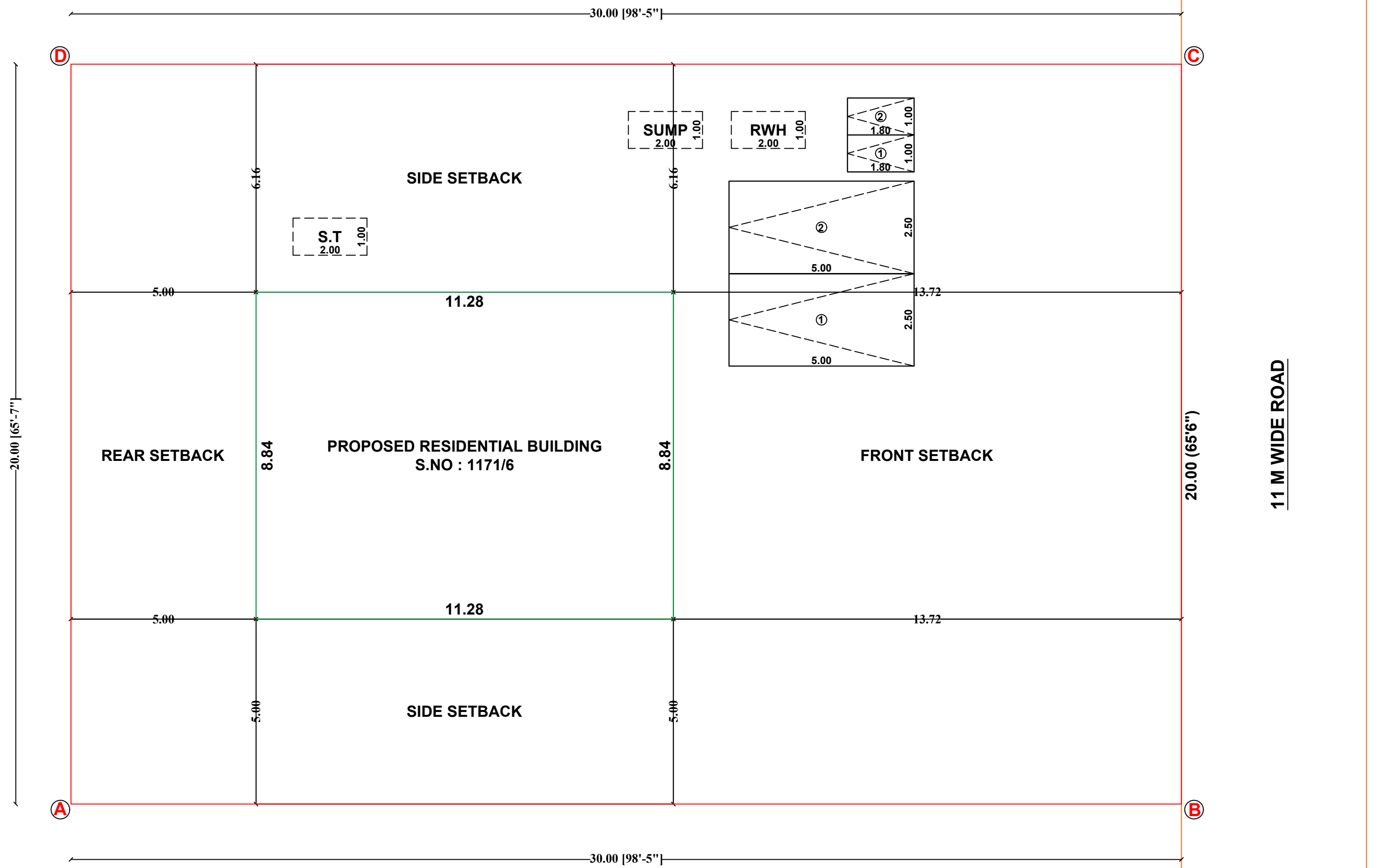
.SITE PLAN.
