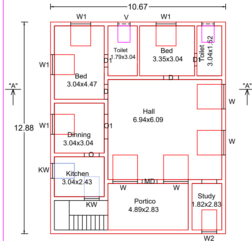
PLAN - G.F
