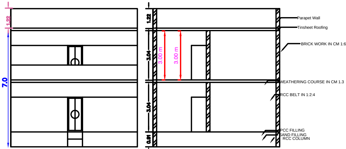
ELEVATION
