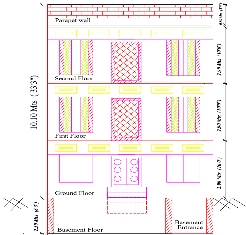
ELEVATION
