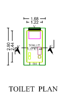
TOILET PLAN
