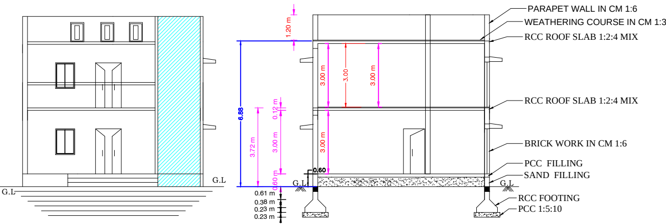
ELEVATION
