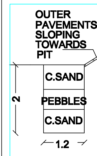
RWH-(N.T.S)
