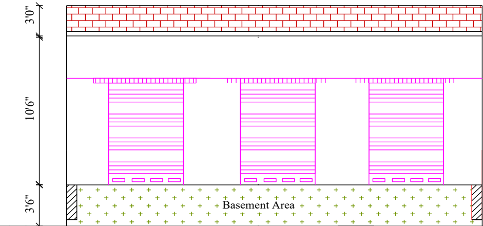
ELEVATION
