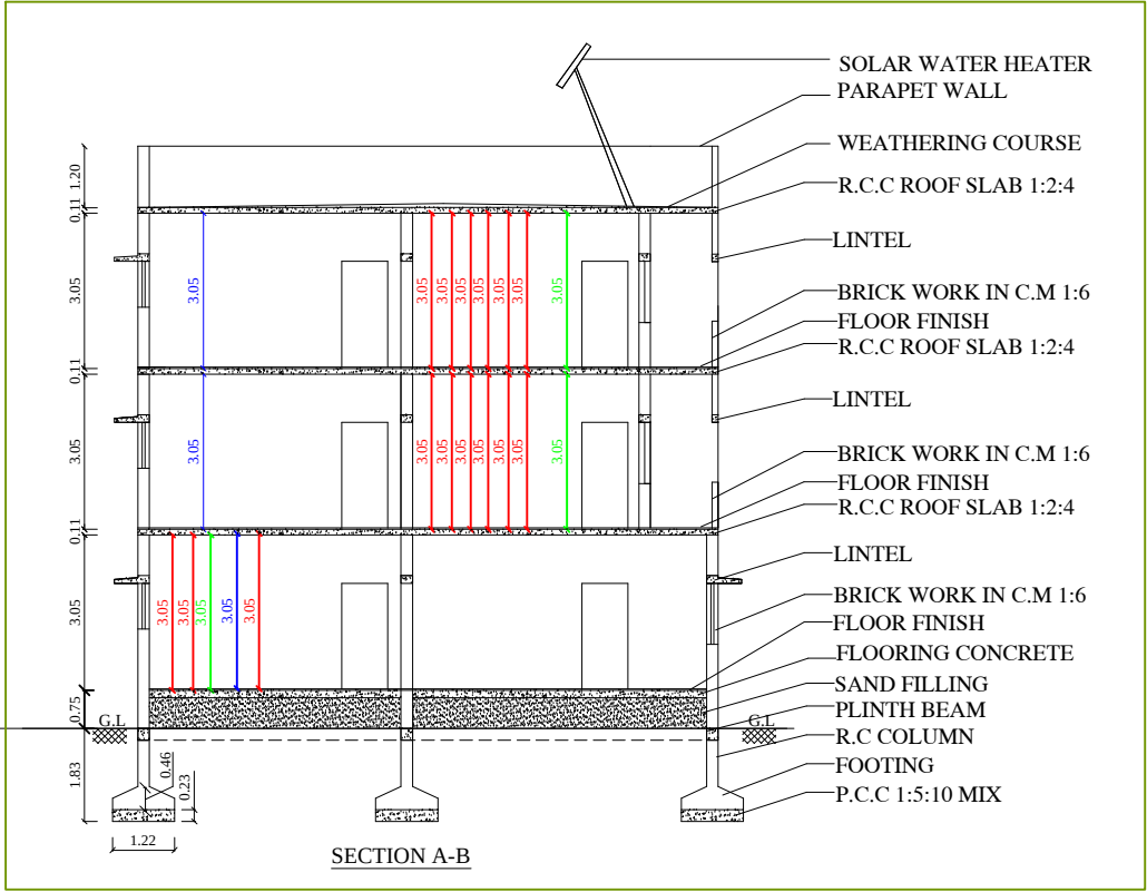
SECTION A-B
