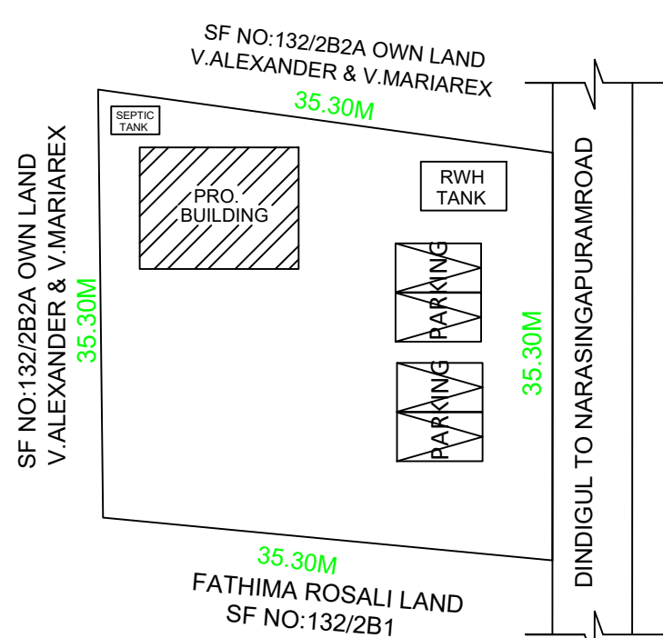
SITE PLAN :
