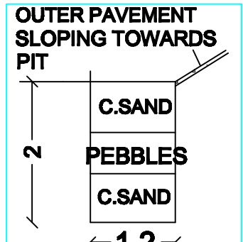
RWH-(N.T.S)
