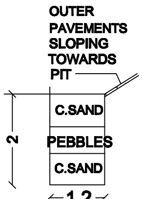
RWH(N.T.S)
