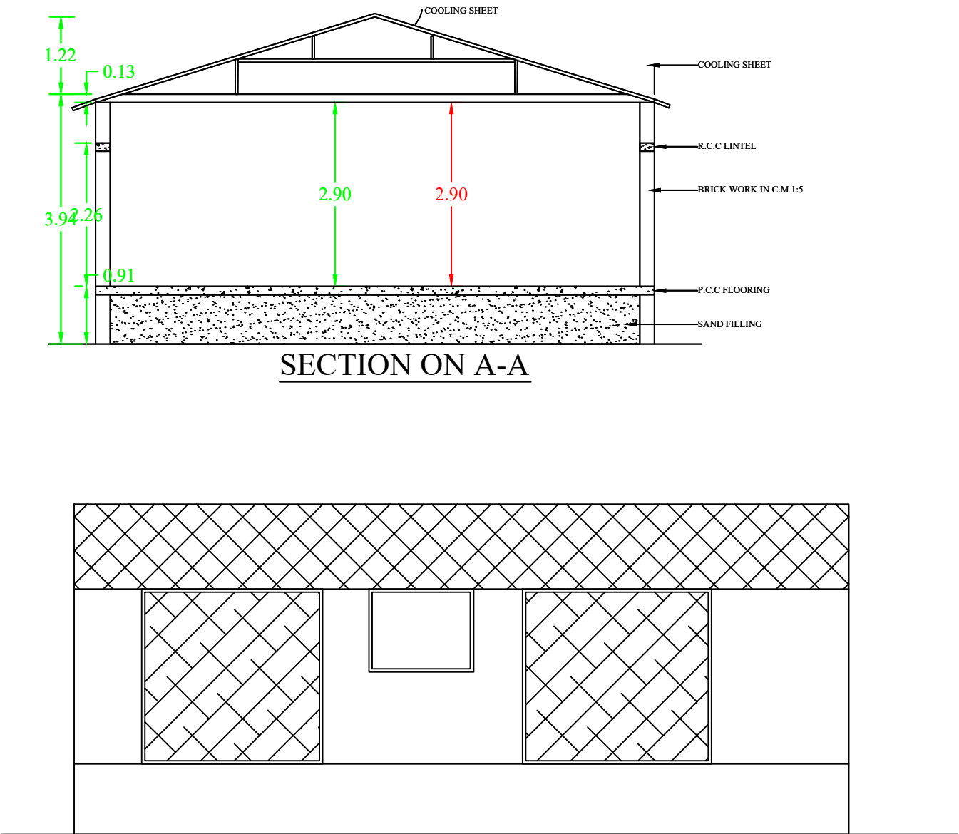
ELEVATION
