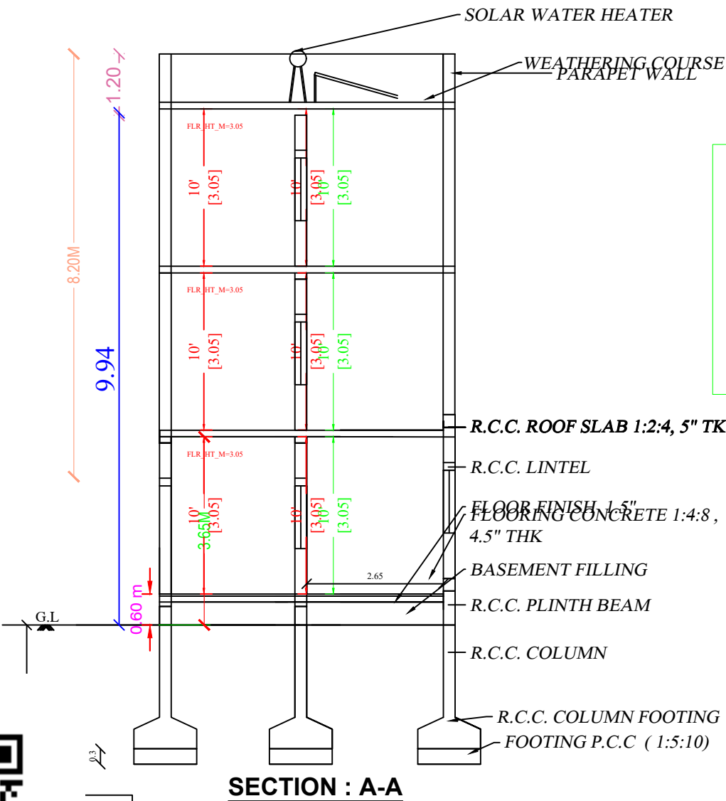
SECTION : A-A
