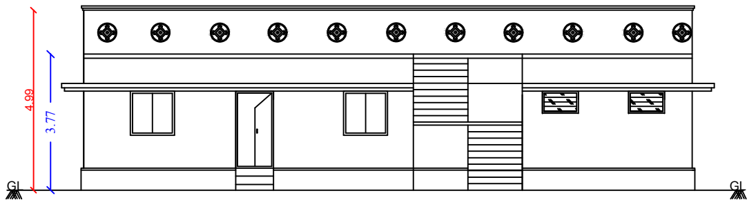
ELEVATION
