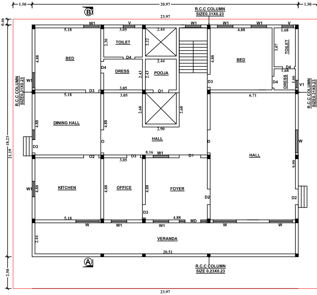
. PLAN .
