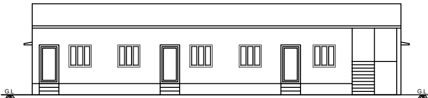
ELEVATION
