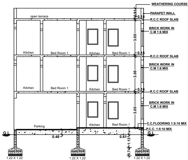
.Section AB.
