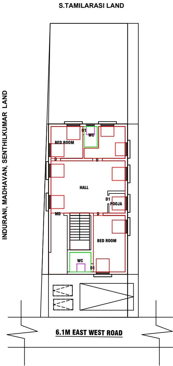
SITE PLAN:
