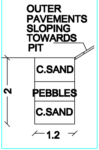
RWH-(N.T.S)
