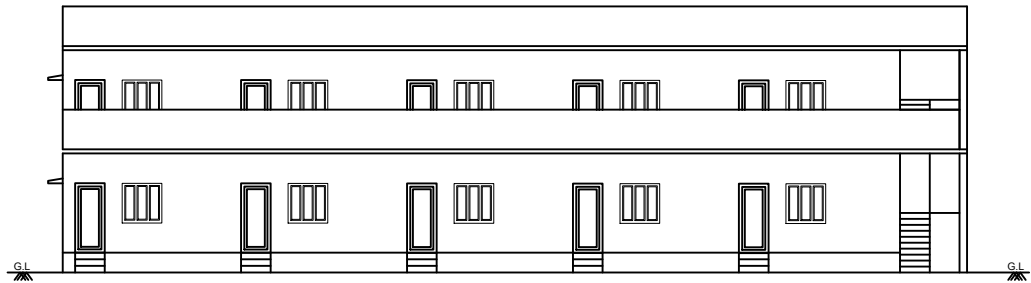
ELEVATION
