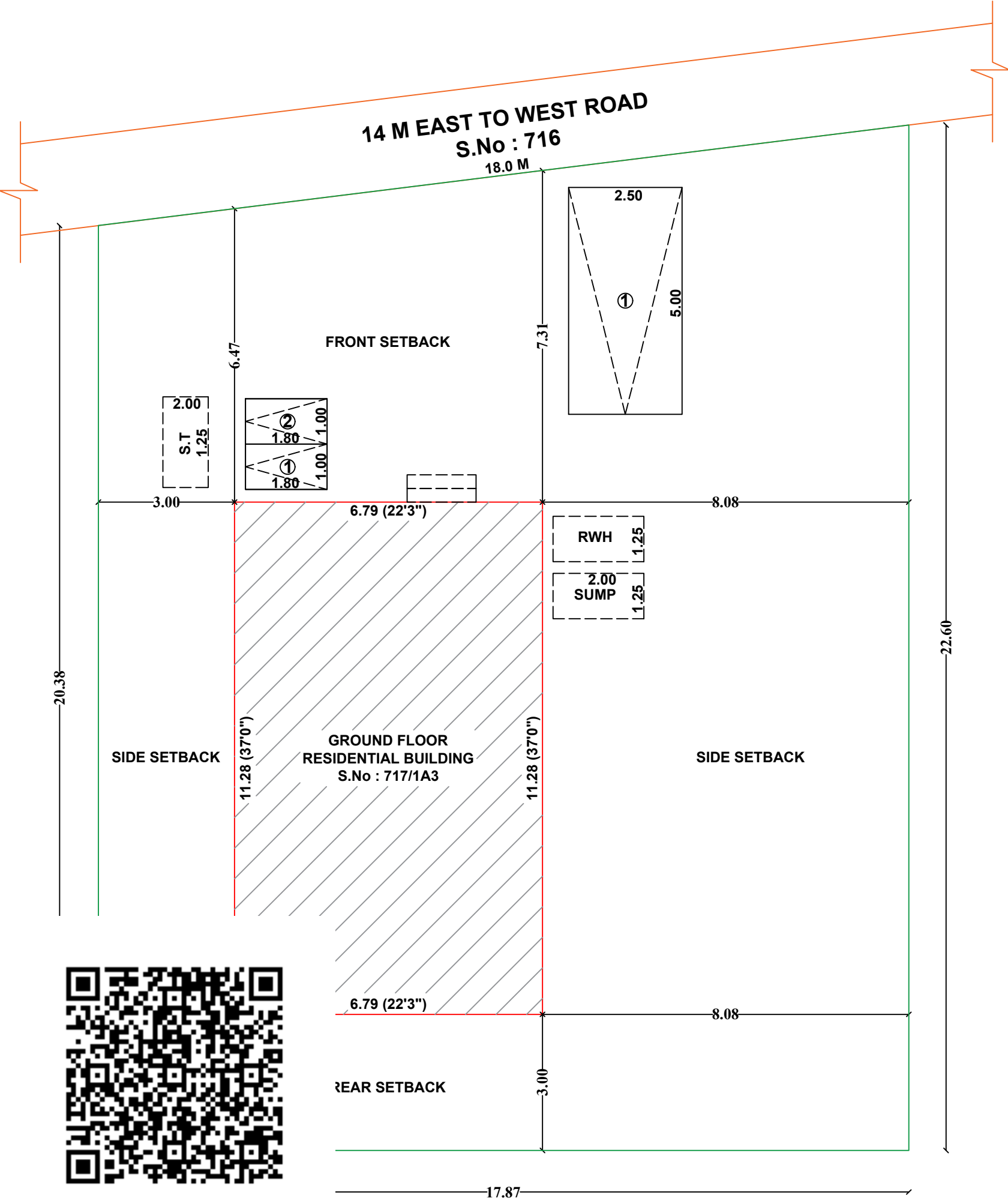
.SITE PLAN.
